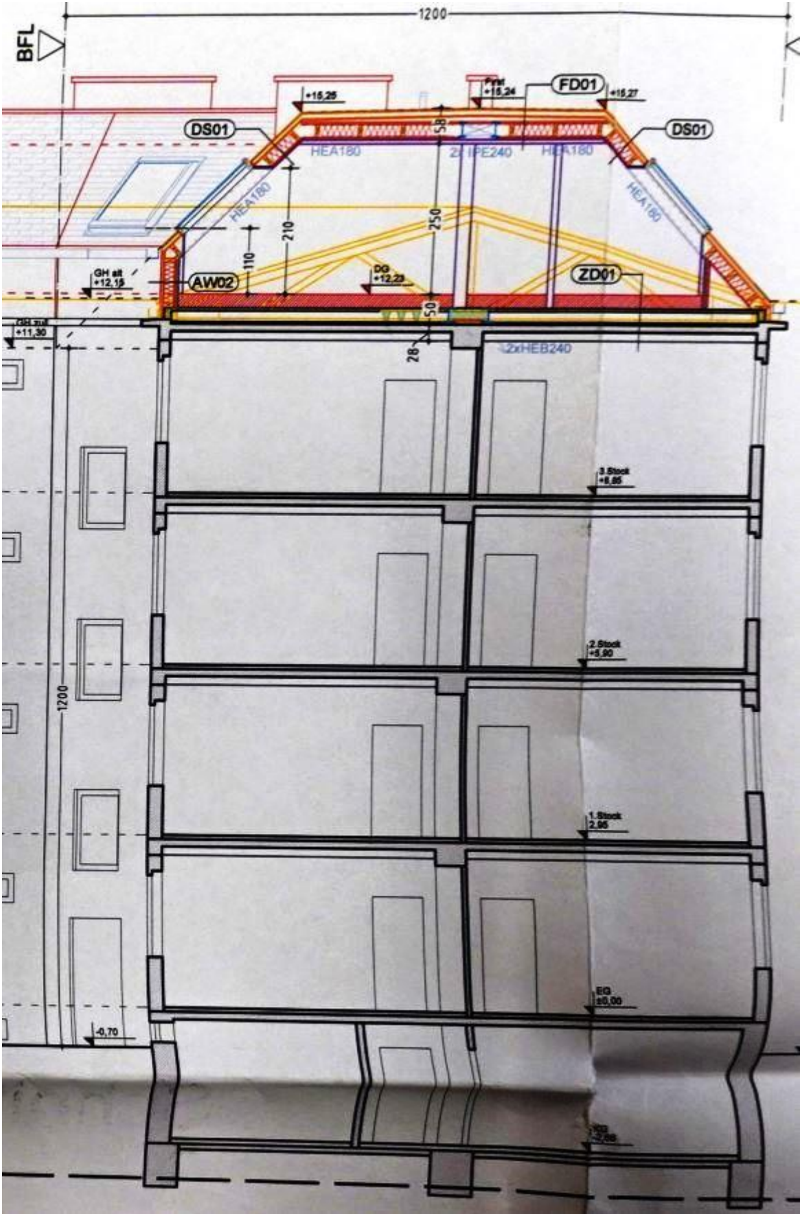
Schnitt B-B
