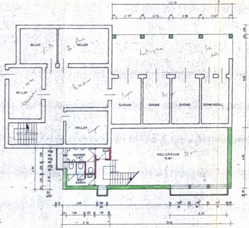
KELLERGESCHOSS
