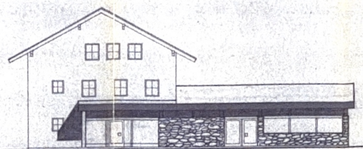
NORD-UND STRASSENANSICHT
