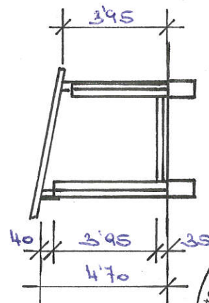
SCHNITT
