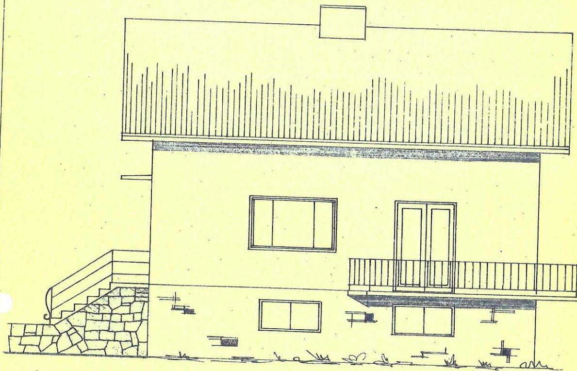
SÜDANSICHT ERDGESCHOSS
