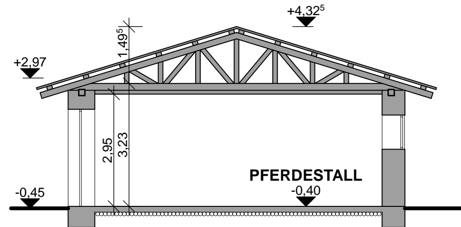
SCHNITT 2-2
