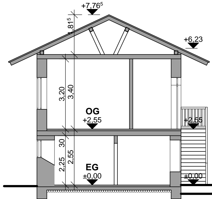
SCHNITT 1-1
