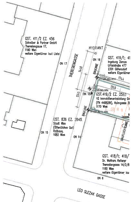
LAGEPLAN M1:500
