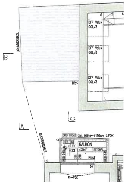
ZWISCHENGESCHOSS
