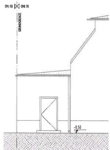
SCHNITTANSICHT A
