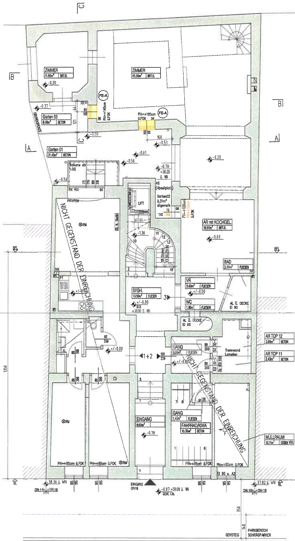
ERDGESCHOSS | M 1:100
