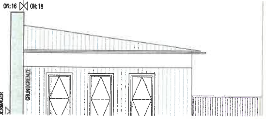
SCHNITT B-B | M 1:100
