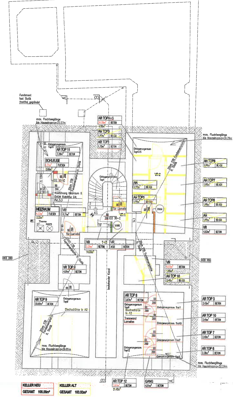
GRUNDRISS - KELLER
