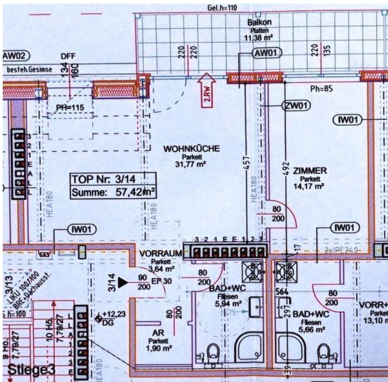
Grundriss Wohnung Stiege 3 Top 14
