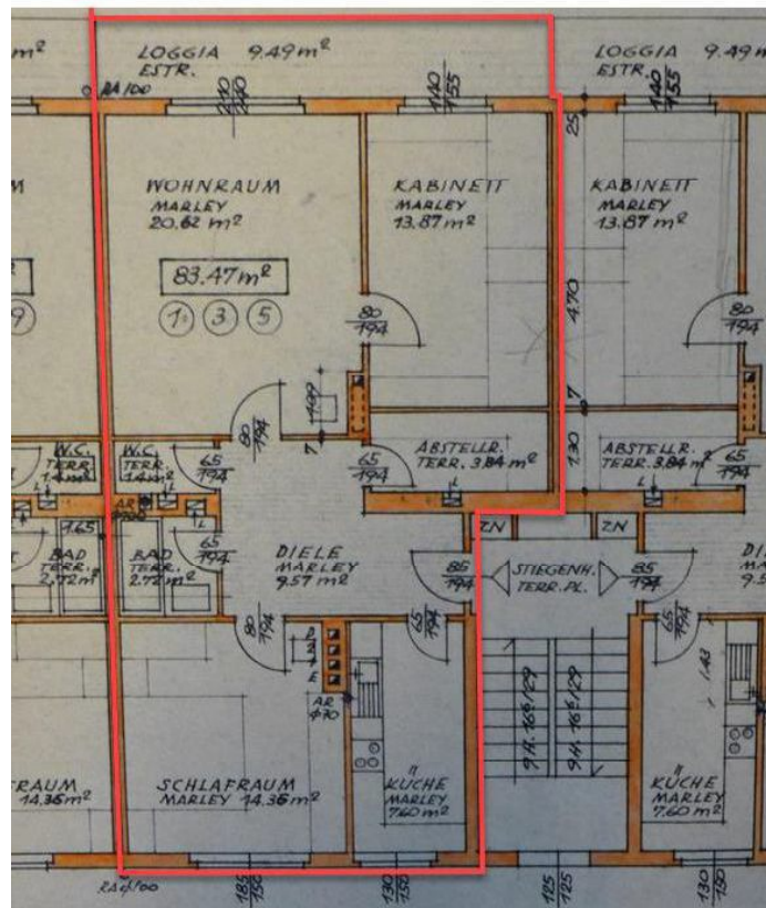
Auswechslungsplan vom 29.08.1961 (auszugsweise)
