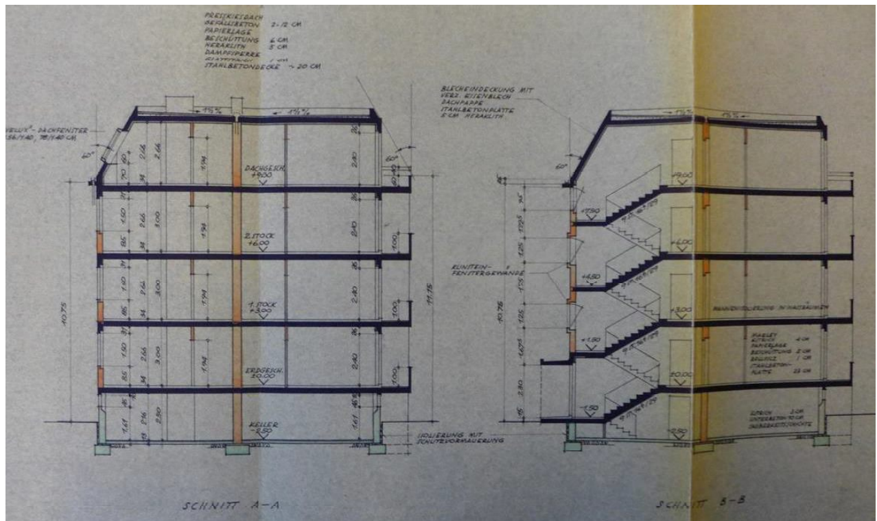
Schnitt A-A, Schnitt B-B Haus I-IV (Auswechslungsplan 08/1961)
