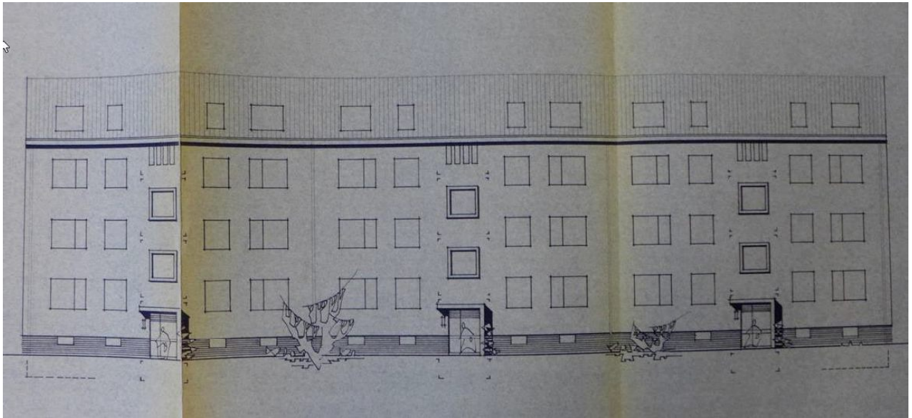
Ansicht Nord Haus I-IV (Auswechslungsplan 08/1961)
