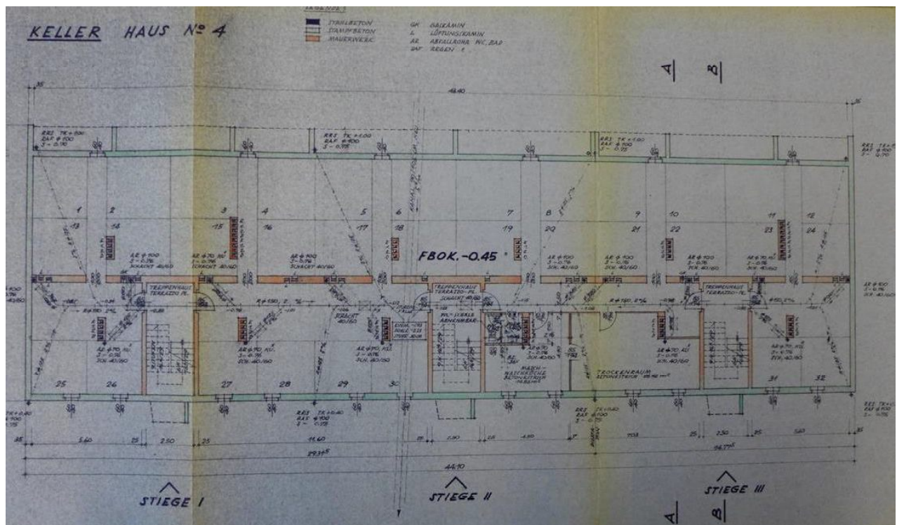
Grundriss Keller Haus IV (Auswechslungsplan 10/1961)
