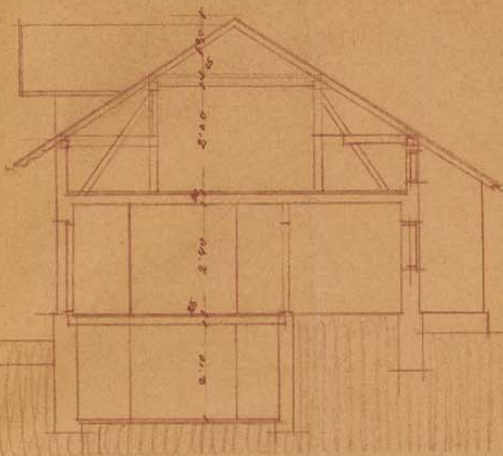
Querschnitt
