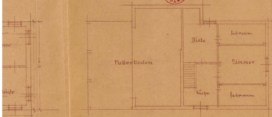
Dachgeschoss
