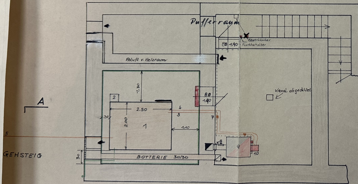
GRUNDRISS
