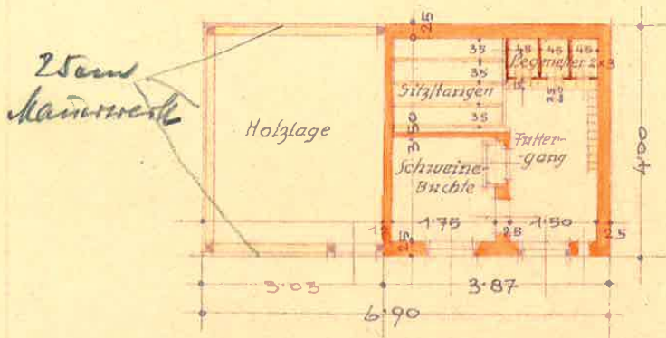
Grundriß
