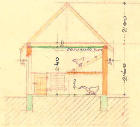
Schnitt
