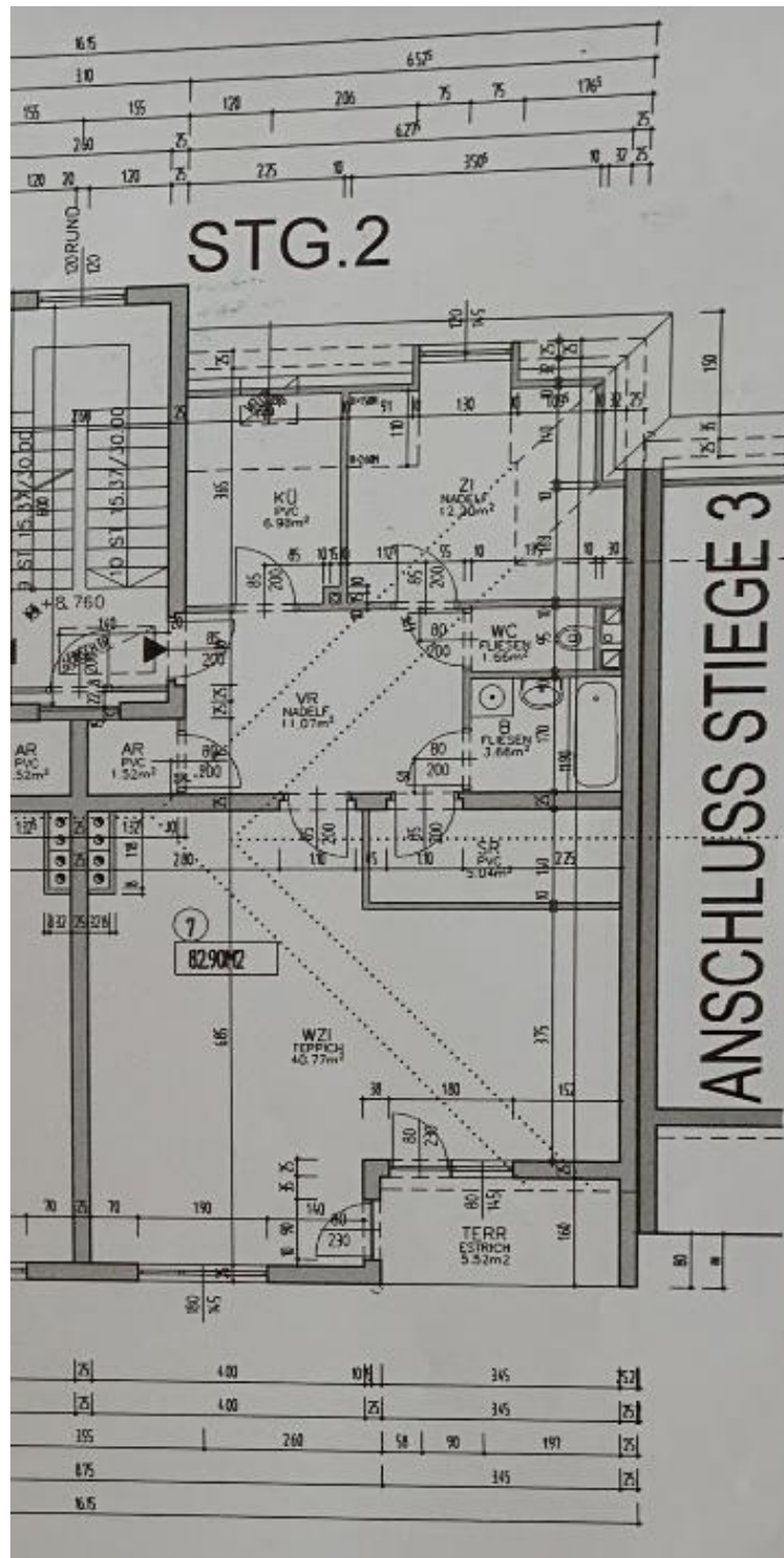
Grundriss W 7 Stg 2
